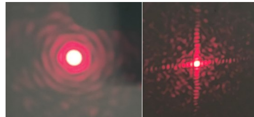
Diffrazione di un laser da un'apertura circolare e da un'apertura quadrata.
